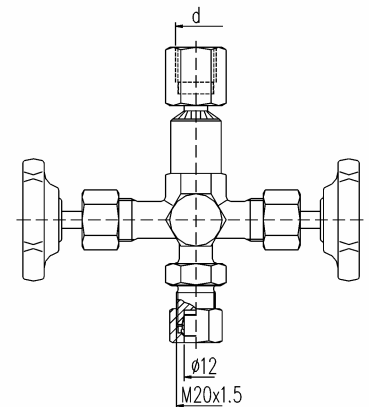
Form B mit drehbarer Muffe und Schaft für Meßgerätehalter
