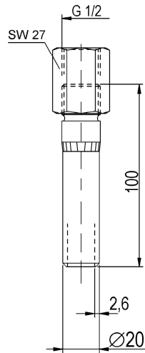
Tube droit
